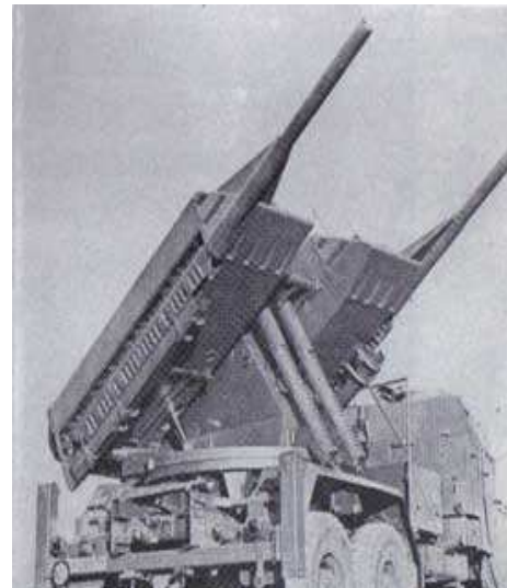
Das Waffensystem der Fa. Oerlikon
